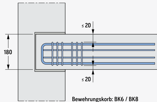
Bewehrungskorb: BK6 / BK8
