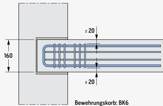
Bewehrungskorb: BK6
